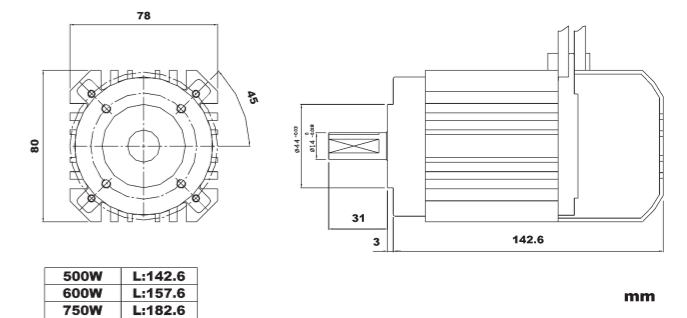
Motor / 馬達
