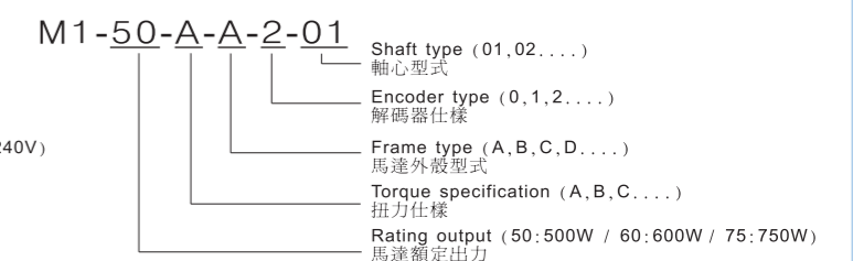
Motor / 馬達
